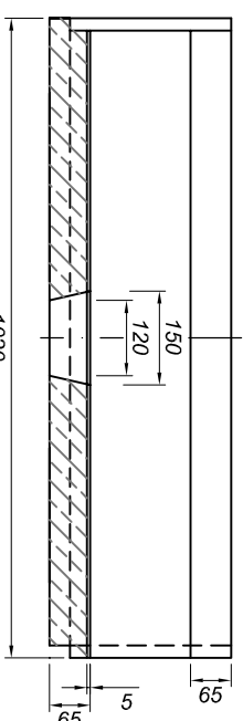
Schnitt B-B
